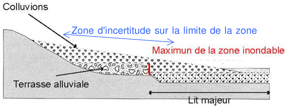
Figure 4 : Colluvions sur lit majeur
