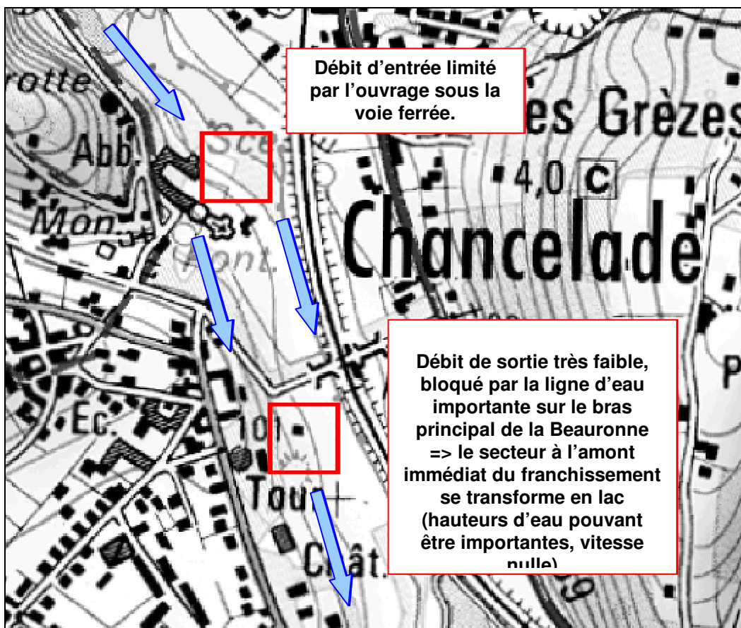
Figure 6 : Schéma de fonctionnement en crue de la Beaunonne et de son bras de décharge à Chancelade
